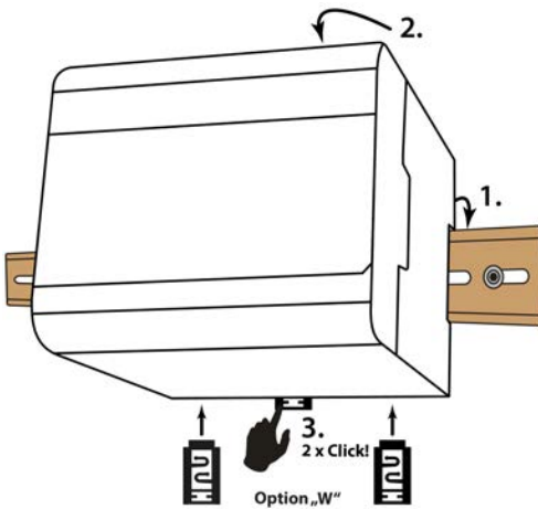
Abbildung 3-4: Montage auf Hutschiene
