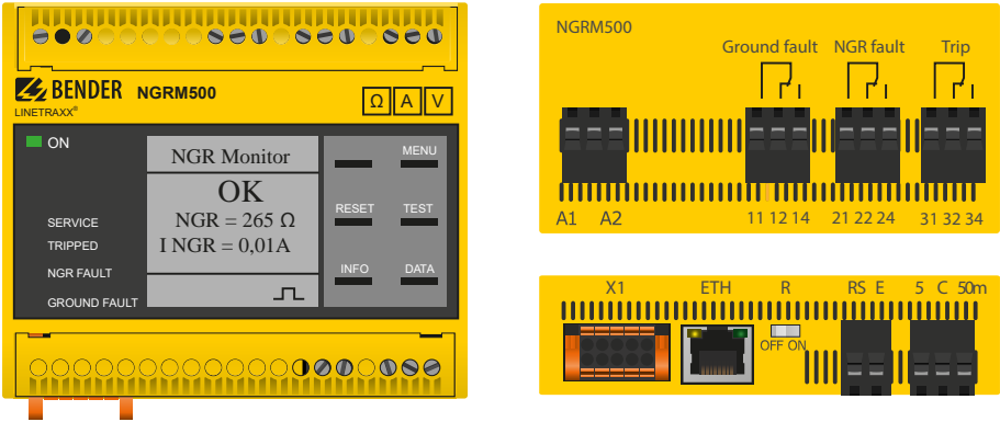
Abbildung 3-2: Gehäuseansicht: Front (links), Oberseite (rechts oben), Unterseite (links unten)
